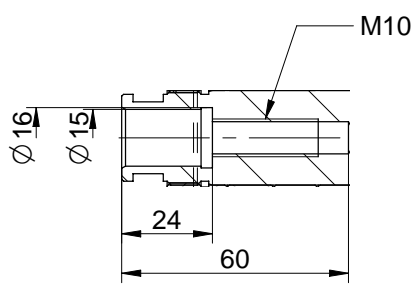
CORTE A-A
