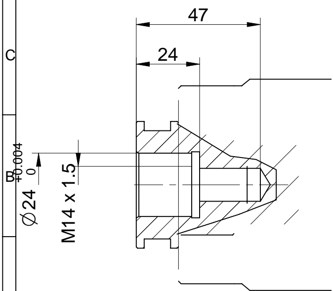
CORTE B-B
