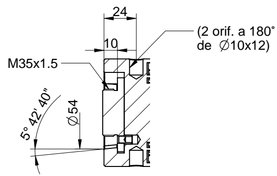
CORTE C-C
