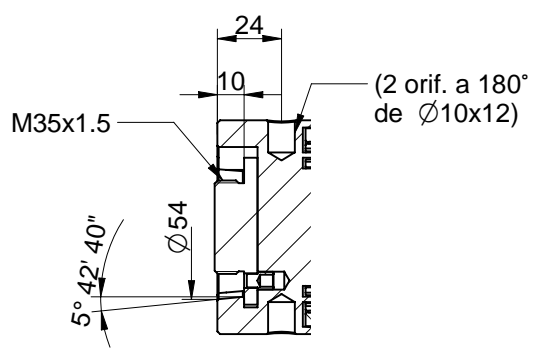
CORTE B-B
