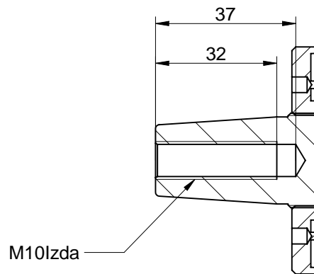
CORTE B-B
